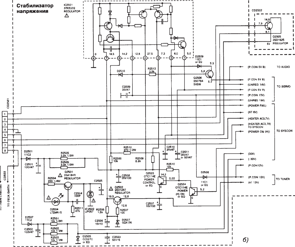
Принципиальные схемы источника питания видеомаягнитофонов VH-300RC/630/730/888/4010/530/2966/821: трансформаторного блока (а) и блока стабилизаторов напряжения (б)
